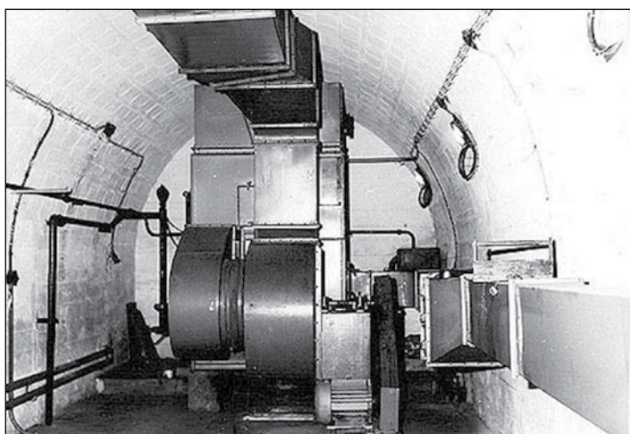
Klimatizační ventrál se dvěma ventilátory středního výkonu.
